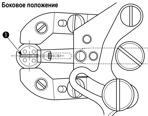
Боковое положение
